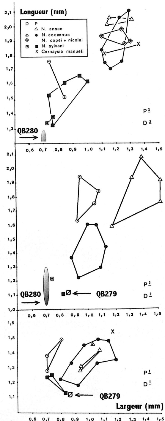
Figure 2 : Diagrammes de dispersion (Longueur x largeur) des P1/, P2/, P3/, D1/, D2/ et D3/ supérieures des Multituberculés paléocènes de Cernay (France), modifiés d'après Vianey-Liaud, 1986 et complétés par les valeurs de QB279 et QB280, limite Paléocène-Eocène de Dormaal (Belgique).
